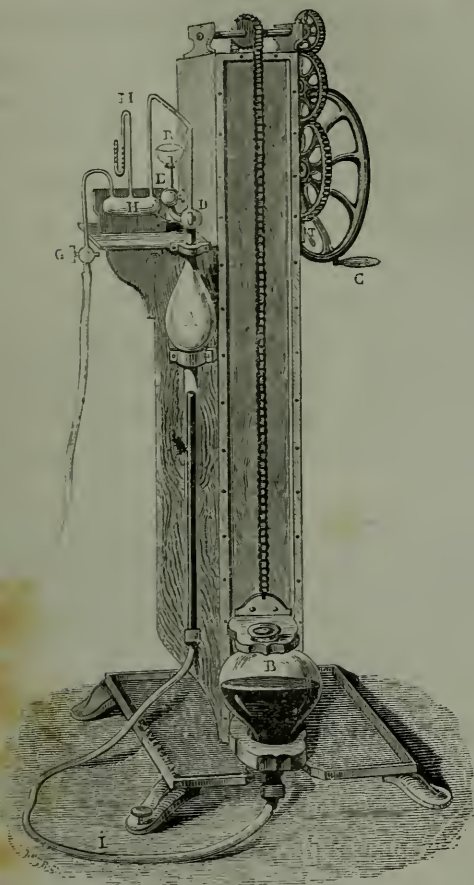
FIG. 66 - Pompe à mercure.
